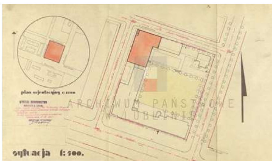
Ryc. 8. Szkoła Budownictwa przy Al. Długosza, proj. S. Łukasiewicz 1931, sytuacja, za: APL UWL-V-WKB, sygn. 1489, kopia projektu za zgodą Archiwum Państwowego w Lublinie
