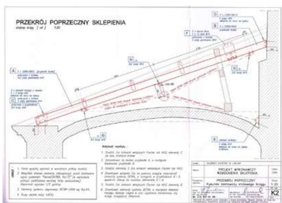
Ryc. 9. Rysunek projektu wzmocnienia sklepienia i więzby dachowej nad pom. Skarbca w z dokumentacji „Skarbiec w Katedrze Lubelskiej”. proj. dr inż. S. Karczmarczyk, AC Konserwacja Zabytków, Kraków 2005-2006 (proj. wykonawczy z archiwum WKZ)
