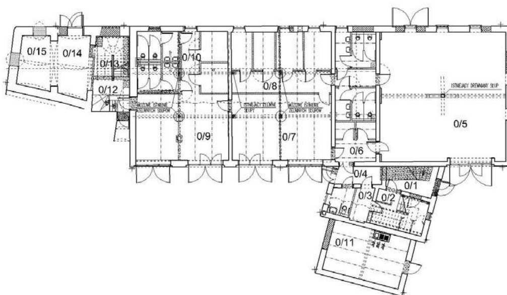
Ryc. 10. Rzut przyziemia; Projekt wykonawczy, Rewitalizacja i adaptacja zabudowań dawnego folwarku (gołębnik) z przeznaczeniem na działalność Dolnobrzeskiego Ośrodka Kultury , główny projektant mgr inż. arch. Jacek Miller, rysunek Małgorzata Doroz-Turek, Wrocław 2011
