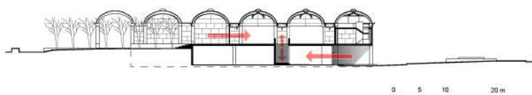
Ill. 3. Musée Kimbell, Fort Worth TX. Version finale, C-Plan . Coupe transversale montrant les deux entrées et la distribution principale.
