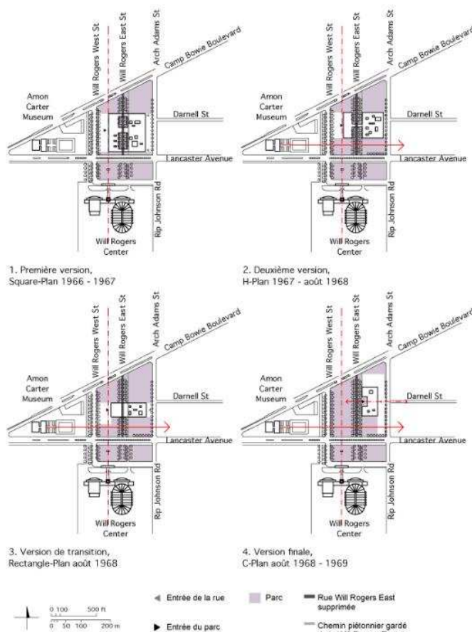
Ill. 2. Musée Kimbell, Fort Worth TX. L'appropriation de l'échelle du site au travers de phases du projet.
