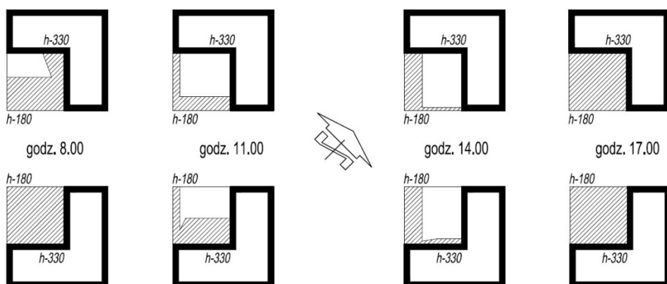
Ryc.13. Przykład zacienienia 21 atrium przy budynku atrialnym typu „L” , w 2 wersjach ułożenia względem stron świata, w godz. 8.00, 11.00, 14.00 i 17.00. Dla uproszczenia wykresów przyjęto: teren jako płaski, wysokość ścian domu – 3.30m, wysokość, ogrodzenia – 1.80m. Cień rzucany tylko przez budynek oraz ogrodzenie leżące na działce (nie uwzględniono terenów sąsiednich);
