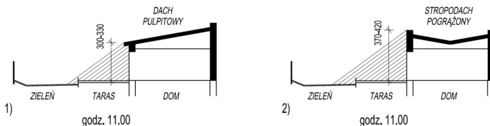
Ryc.14. Przykład zacienienia atrium o godz. 11.00 przy budynku zadaszonym 1) dachem pulpitowym oraz 2) dachem pogrążonym;
