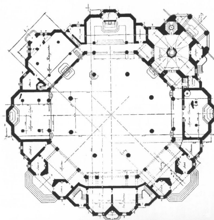
Ryc. 6. Kościół p.w. Św. Rocha, rzut na poziomie nawy głównej, arch. Oskar Sosnowski (1927-1946)
