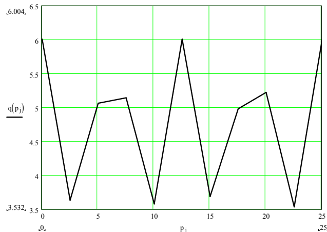
Рис. 4. Втрати гички ( q , %) в залежності від значень зсуву фаз ( P , см) косинусоїди коливань гичкорізального апарату відносно косинусоїди нерівностей поверхні ґрунту ( H = 3,7 \text{ см} )
