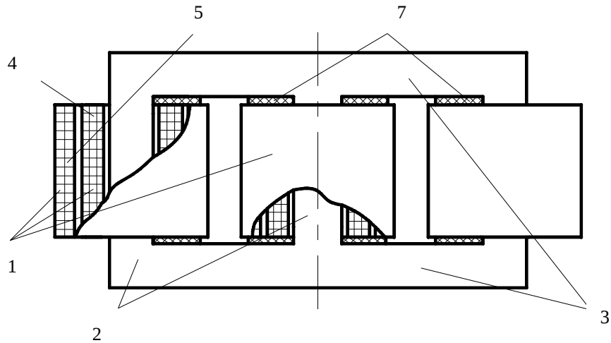
Рис.1. Активная часть индукционного устройства
