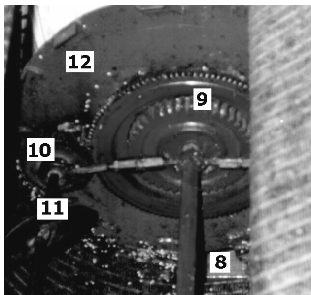
б) привод бичей
