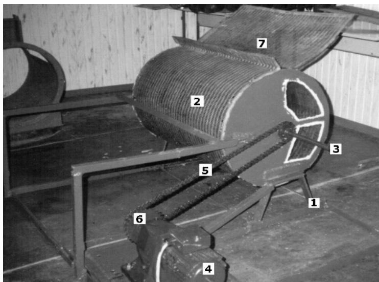
а) общий вид лабораторной установки
