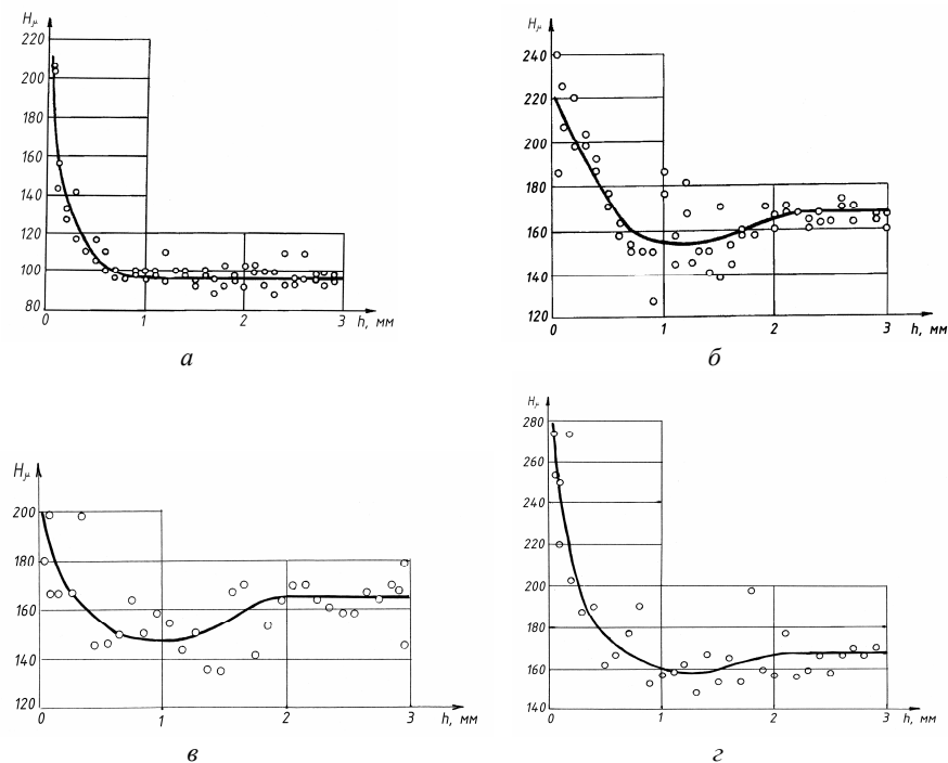
Рис. 3. Распределение микротвердости по глубине упрочненного слоя: а – армкожезецо, r_p = 2,5 мм, P = 1,5 кН; б – сталь 45, r_p = 2,5 мм, P = 4,5 кН; в – сталь 45, r_p = 5 мм, P = 5 кН; г – сталь 40Х, r_p = 2,5 мм, P = 5,5 кН
